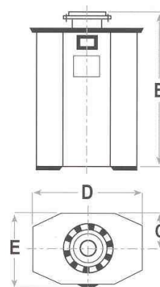
Balgengaszähler G40 – G65
