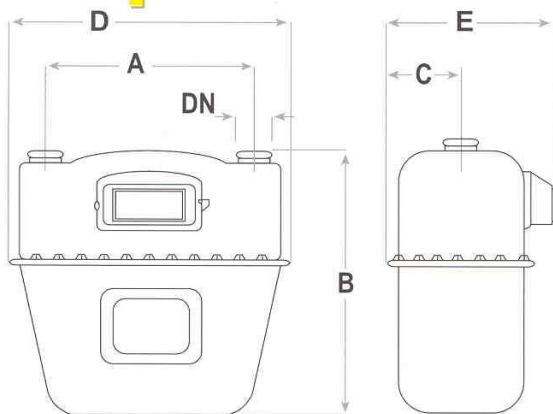
Balgengaszähler G4 – G25
